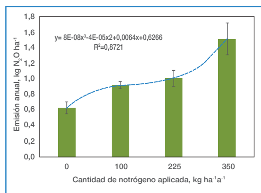
Figura 34. Emisión anual de óxido nitroso determinada con diferentes dosis de nitrógeno aplicado a una plantación de café bajo sombra en Naranjo (A) y, San Marcos de Tarrazú (B), Costa Rica.
